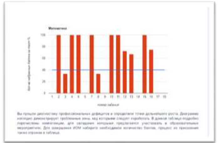
Касьянова С.В.
